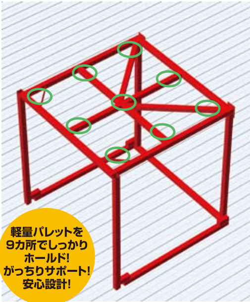
接合部
