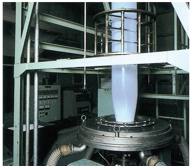
インフレーション押出機
